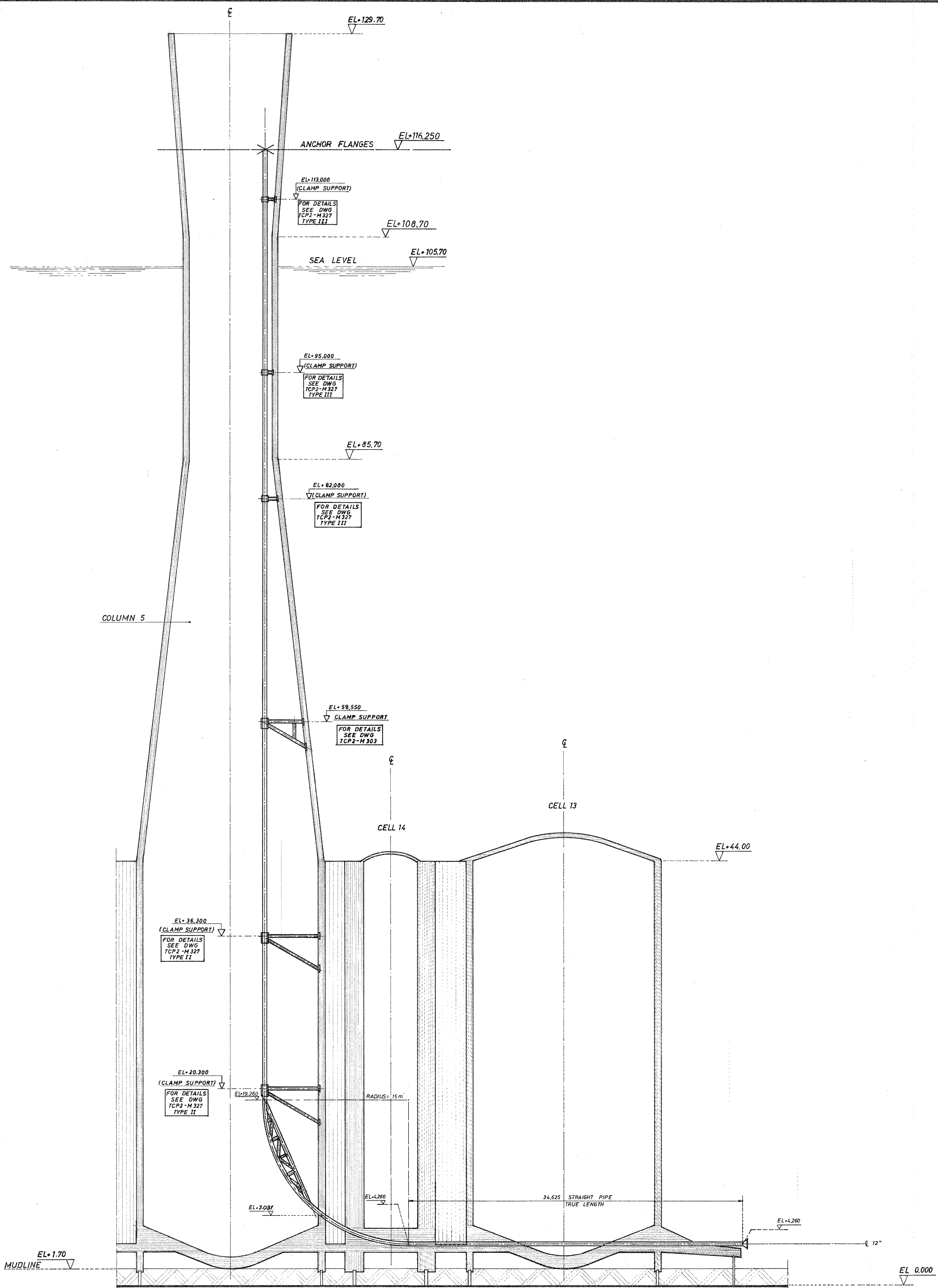
SECTION THRU 12" J TUBE COLUMN 5 N° J6-12
