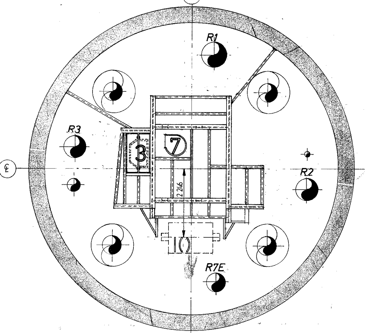
PLAN VIEW EL 109 040 T.O.S.
