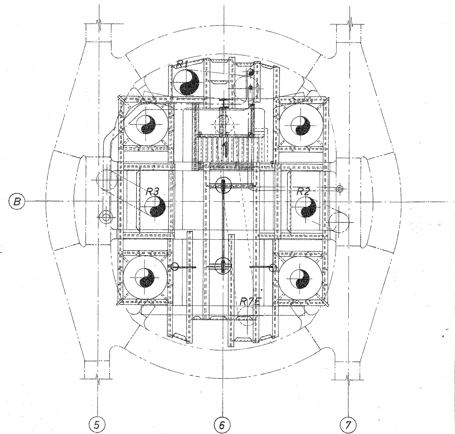
PLAN VIEW EL 131 700 T.O.S.
