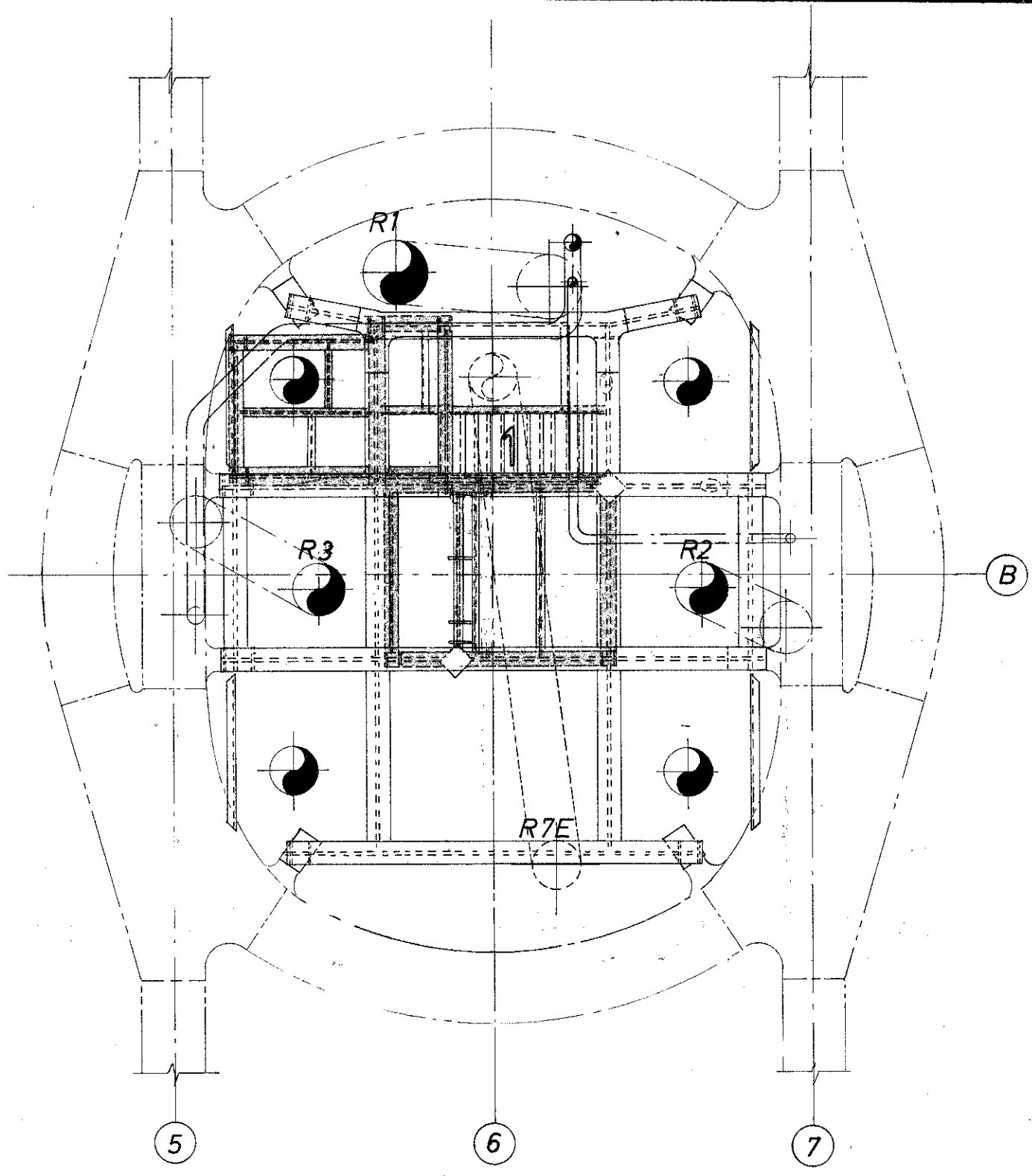
PLAN VIEW EL 131 510 T.O.S.
