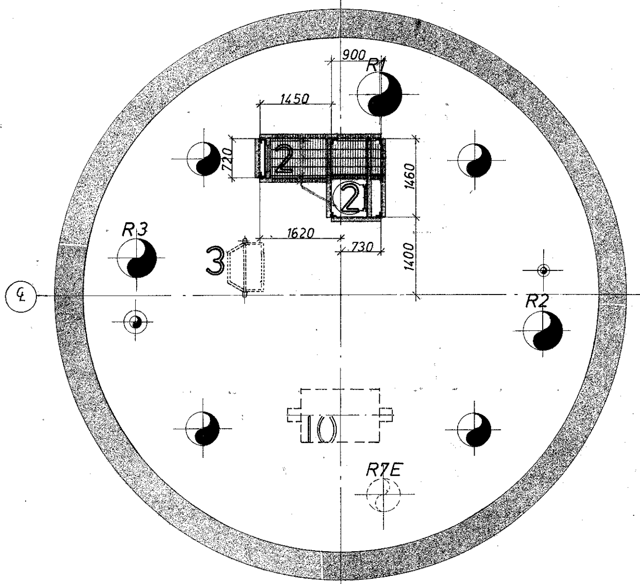
PLAN VIEW EL 124 932 T.O.S.
